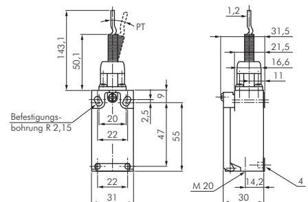
Federstab Edelstahl
