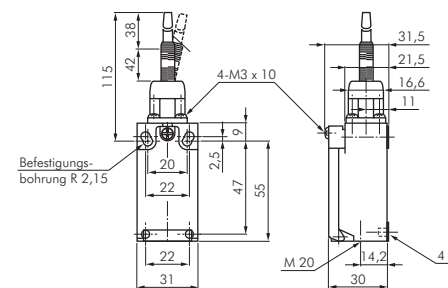
Federstab Kunststoff
