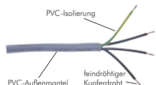
PVC-Außenmantel
